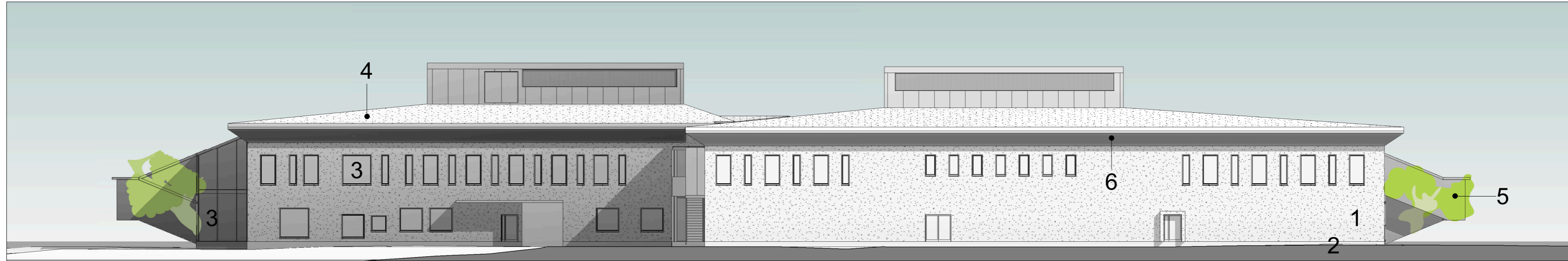
Julkisivu pohjoiseen 1 : 250
